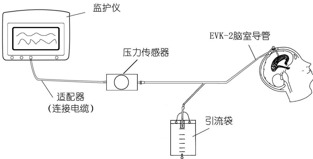
EVK脑室导管和监护仪连接示意图
